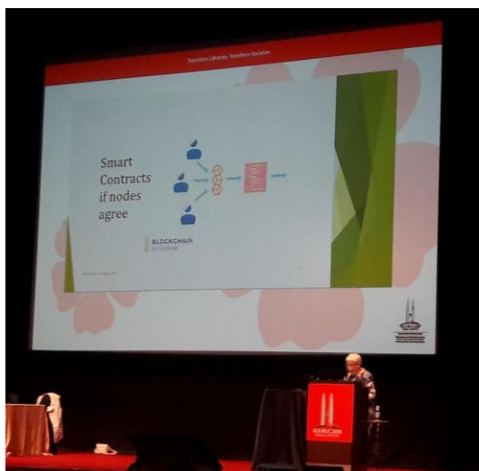
Bild 6 Blockchain
